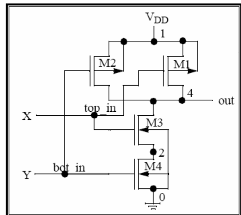
گیت NAND
